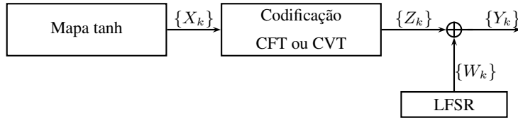
Figura 3.10: Diagrama em blocos do esquema de geração de um PRNG usando seqüências- m .
