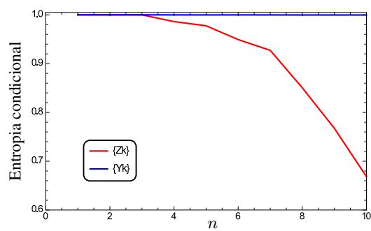
Figura 4.17: Entropia condicional de Z_k e Y_k versus n para mapa e -tanh com r = 3 e q = 3 .
