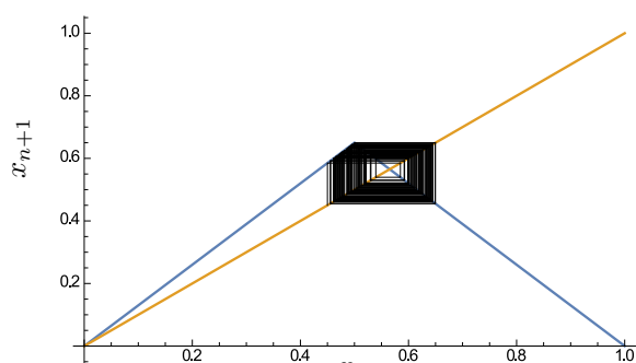
Figura 2.5: Cobweb do mapa da tenda para 1 < \beta < \sqrt{2} .
