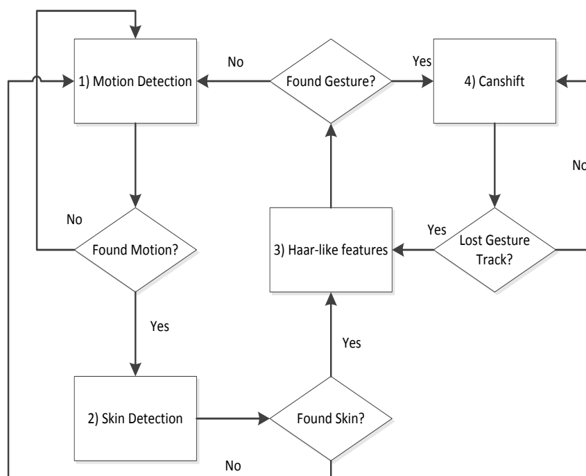
Figura 5.9: Diagrama do processo de reconhecimento de gestos utilizando motion, skin, Haar cascade e CamShift.
