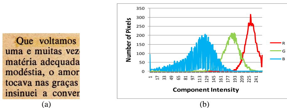
Figura 2.14: (a) Imagem após aplicação do primeiro passo do algoritmo 2.4 (b) Histograma da área afetada pelo marcador amarelo.
