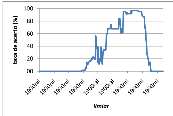
Figura 3.3: Gráfico da taxa de acerto de reconhecimento caracteres com a variação do parâmetro limiar .
