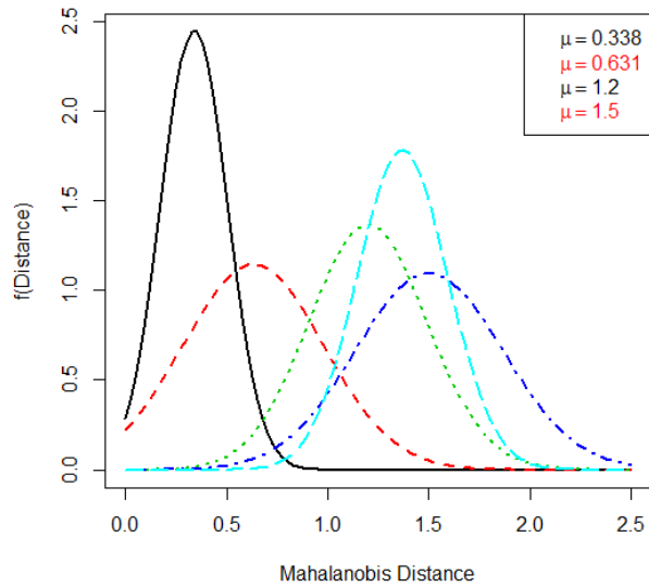
Figura 4.2: Distribuições da marca Bic obtidos da Tabela 4.1, as curva mais a esquerda são comparações entre traços da mesma caneta, a curva vermelha comparações de distâncias entre canetas Bic e as 3 curvas mais a direita são comparações de textos entre Bic e as Marcas FaberCastell, Pentel e Pilot.
