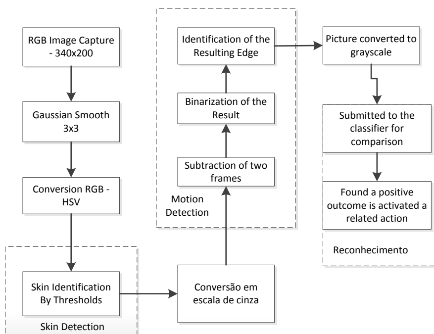
Figura 5.7: Processo de detecção da tonalidade de pele associado ao motion detection.
