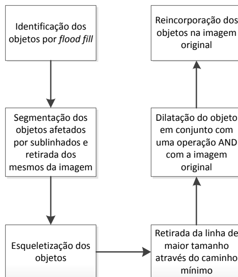
Figura 2.34: Fluxograma do algoritmo proposto para retirada de sublinhados em imagens binarizadas.
