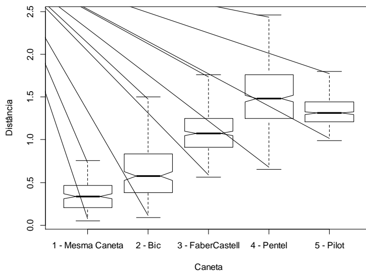
Figura 4.3: Notched Box Plot das distâncias entre os objetos de texto da Marca Bic comparados com as marcas em estudo, as colunas correspondem as distribuições da Figura 4.2.
