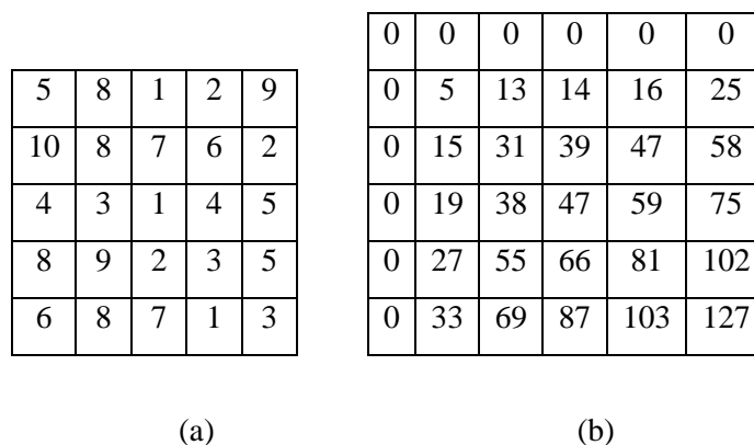
Figura 5.4: (a) Imagem Original. (b) Adição de linha e coluna para cálculo da imagem integral.
