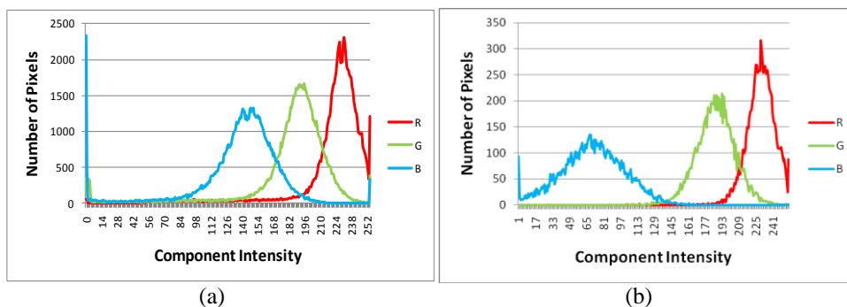
Figura 2.12: Histogramas da imagem 2.4a. (a) Área não afetada pelo selecionador. (b) Área afetada pelo selecionador.
