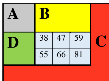
Figura 5.6: Definição das regiões em uma imagem integral.
