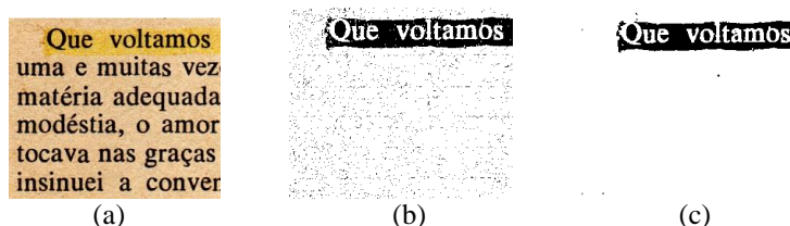
Figura 2.13: (a) Imagem Original. (b) Máscara encontrada pela aplicação do algoritmo de Otsu na componente azul da figura 2.13a sem os pixels do texto. (c) Máscara final com ruído de sal e pimenta filtrado.
