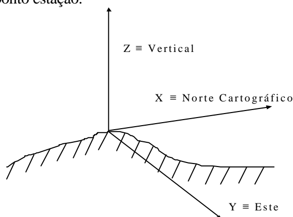
Figura 2.5 - Referencial local, topocêntrico-horizonta
